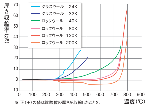
■ 温度と厚さ収縮率の関係※
