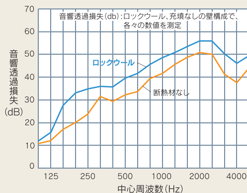
■ 遮音性能比較
