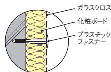
<プラスチックファスナー工法>
