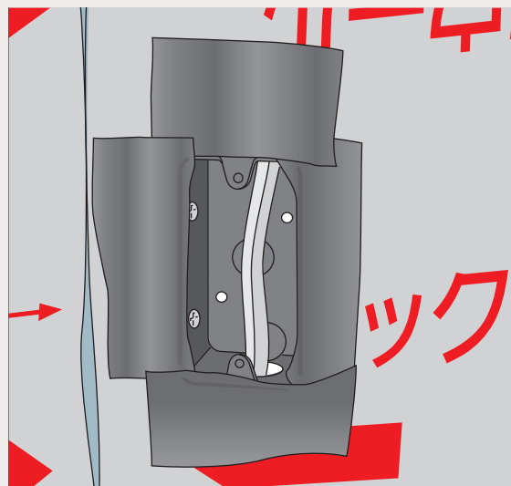
気密テープを用いた場合
