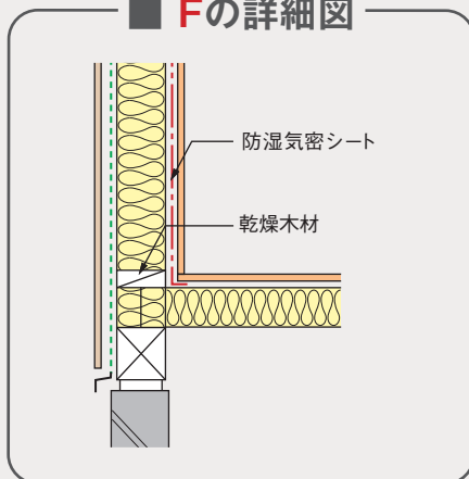
■ Fの詳細図
