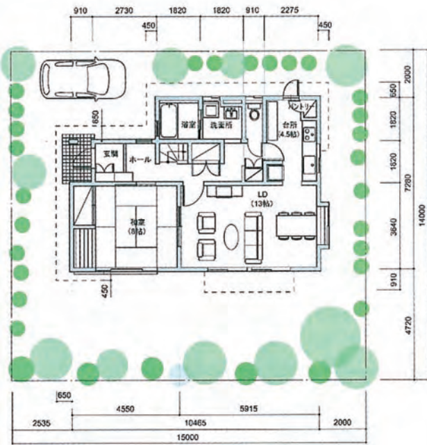
■1階平面図
