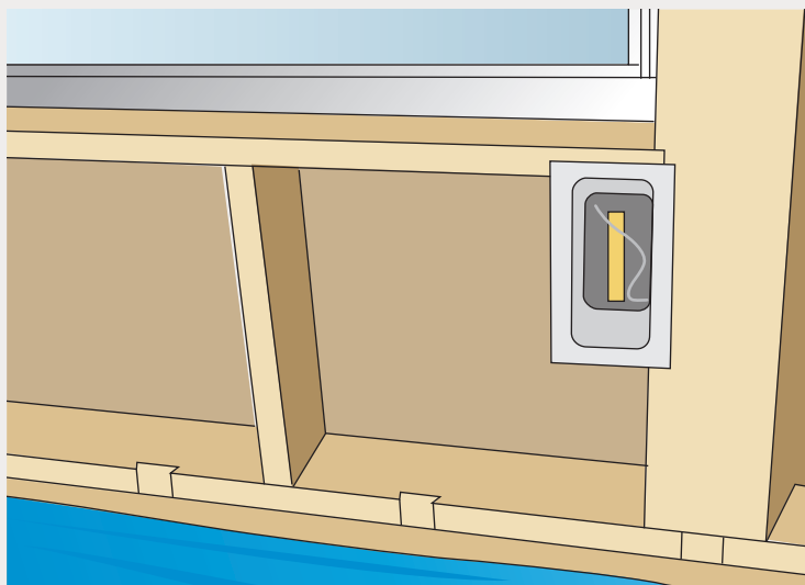
専用部材を用いた場合
