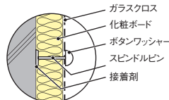
<ピンボタン工法>
