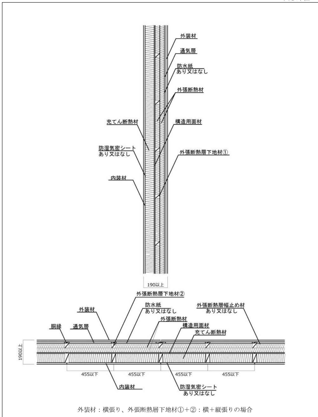
図 4 構造説明図
