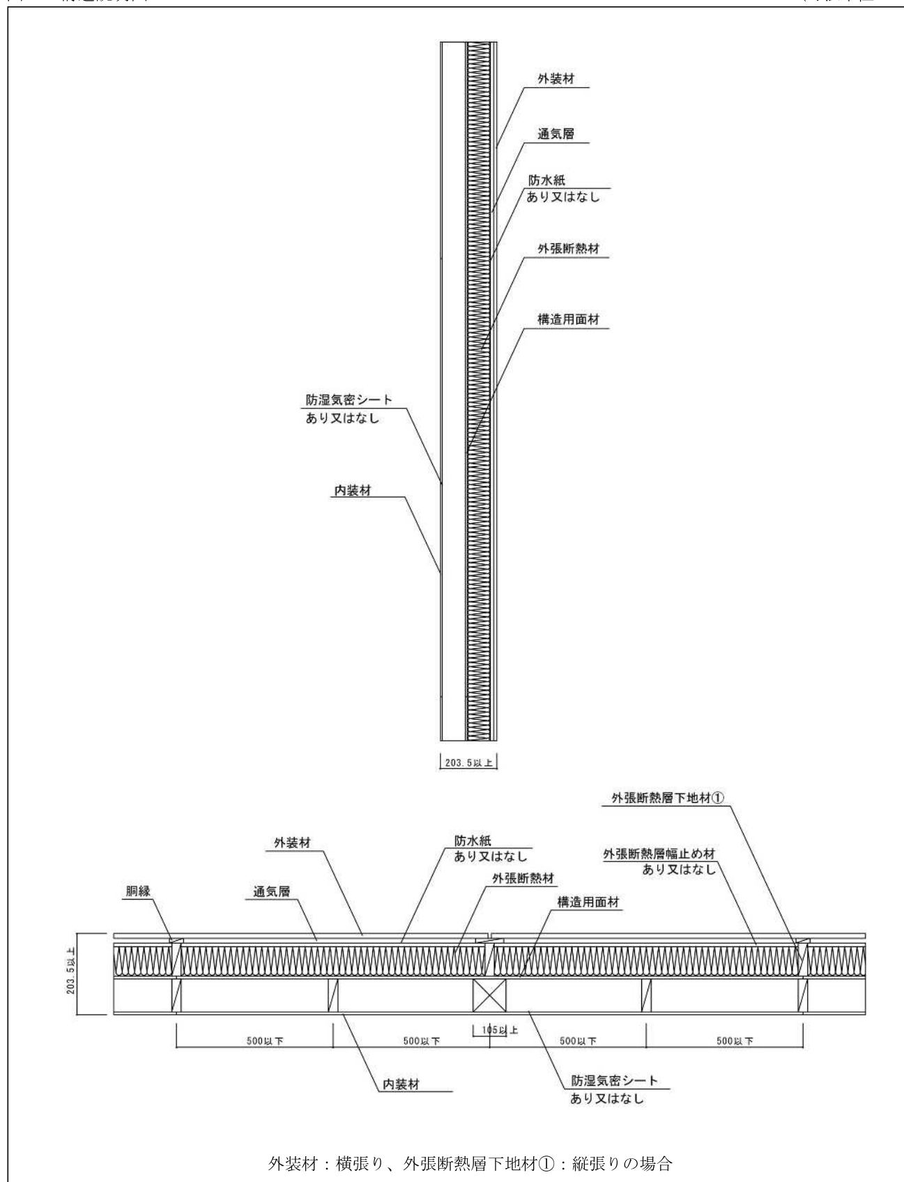
図3 構造説明図
