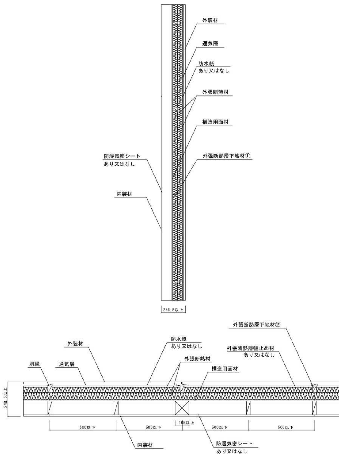
図4 構造説明図
