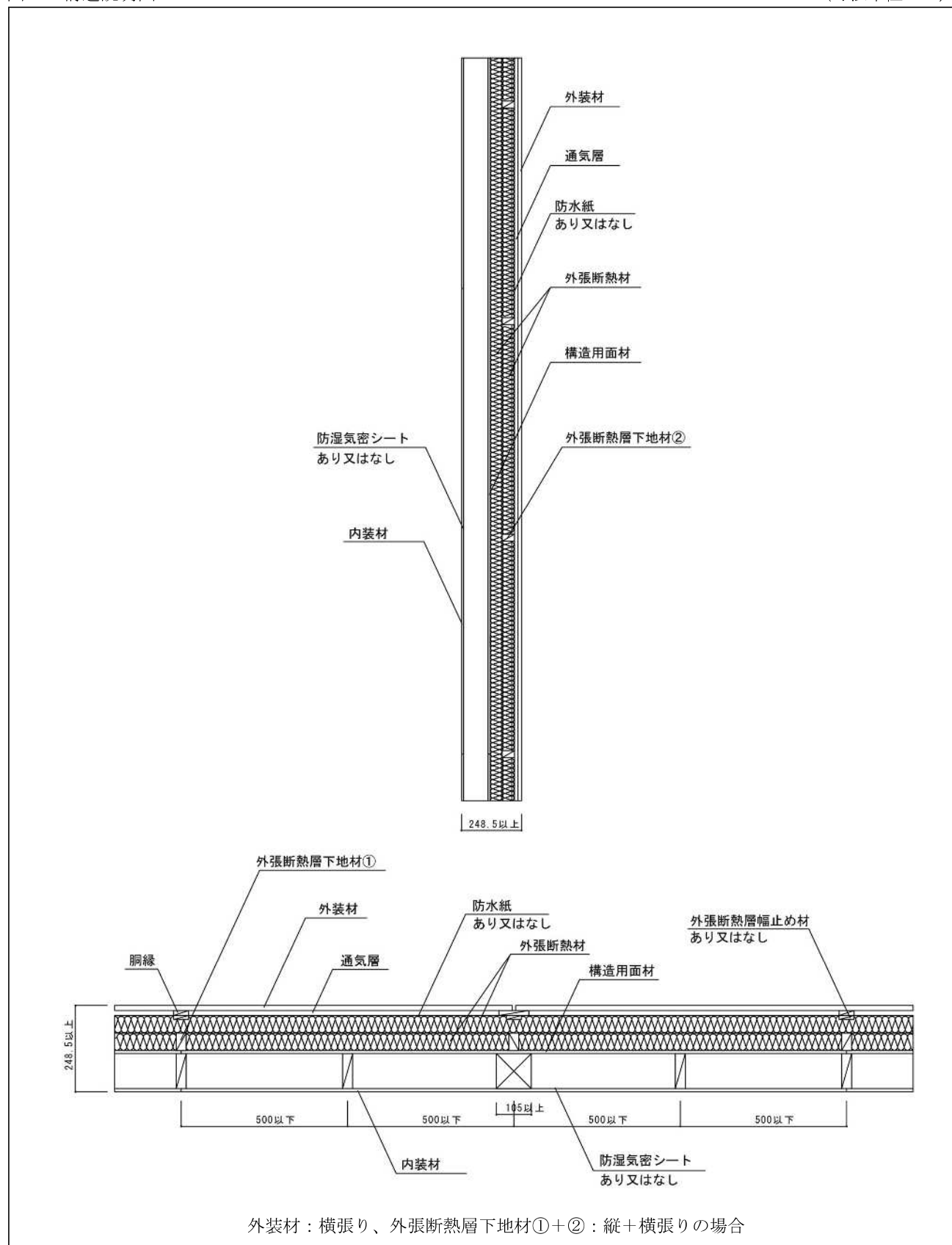
図5 構造説明図
