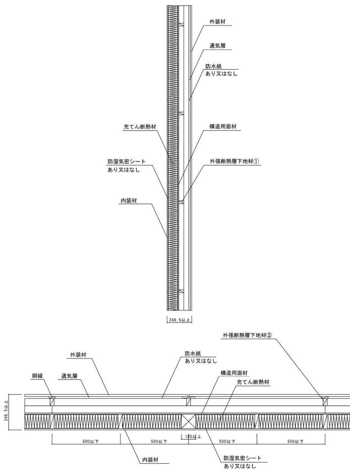
図 4 構造説明図
