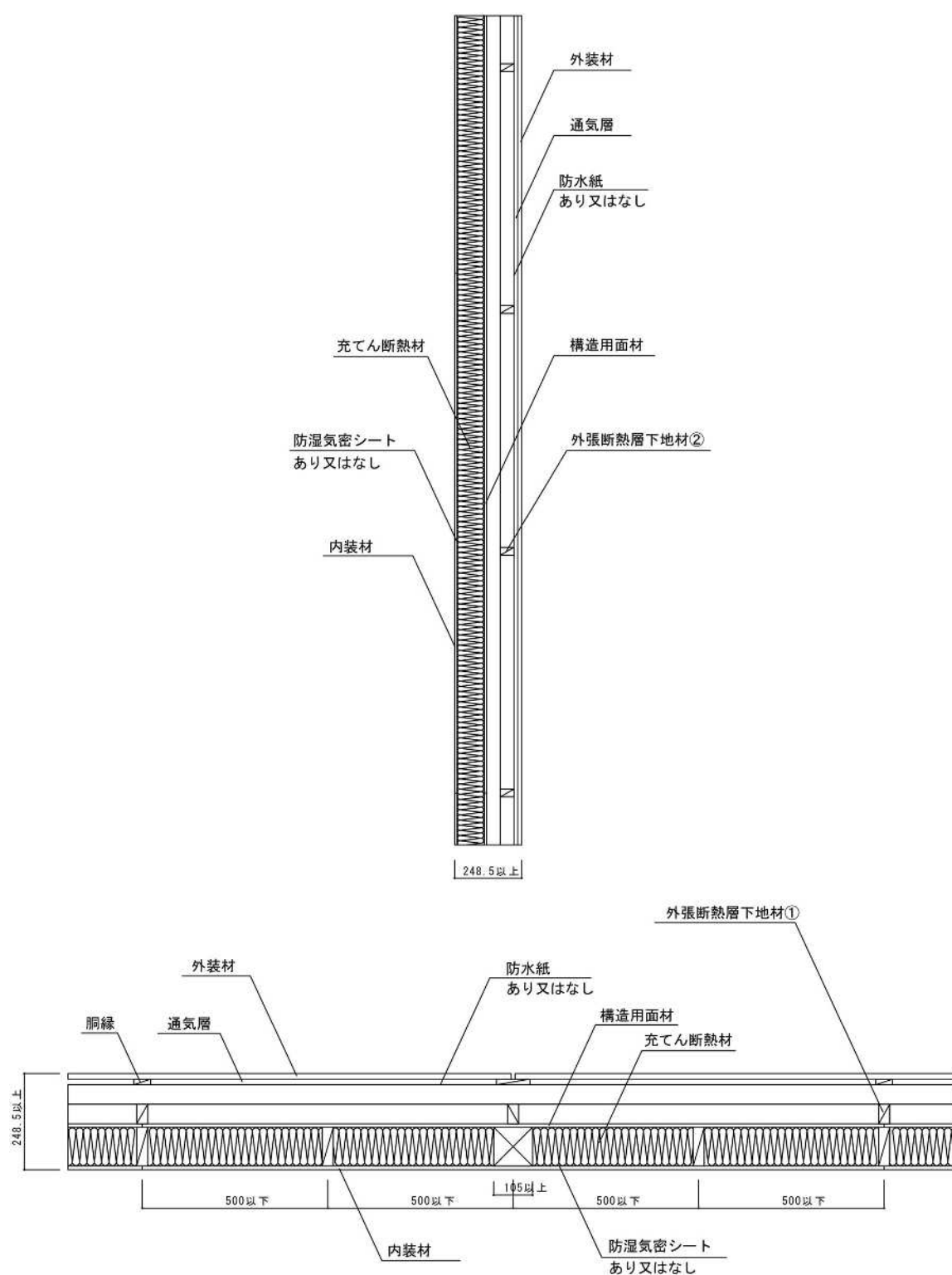
図5 構造説明図
