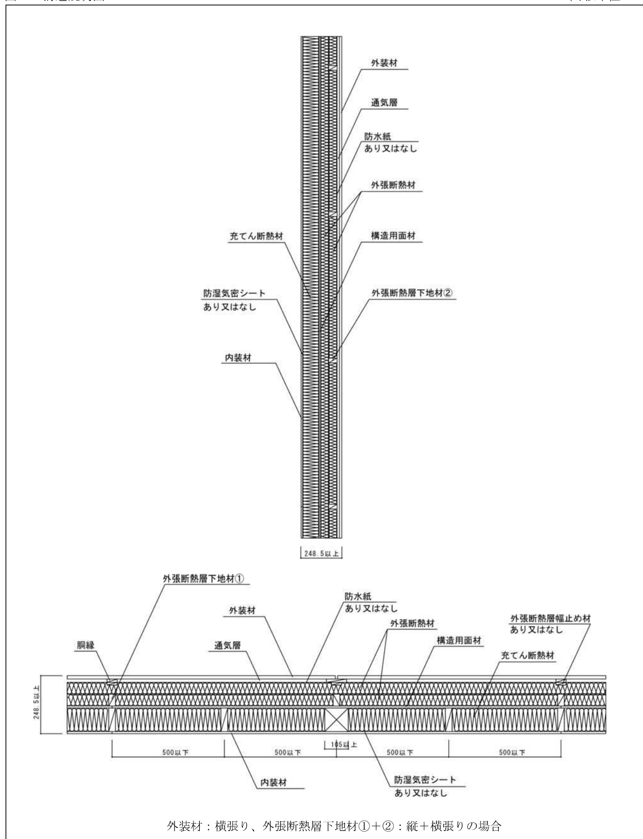
図5 構造説明図
