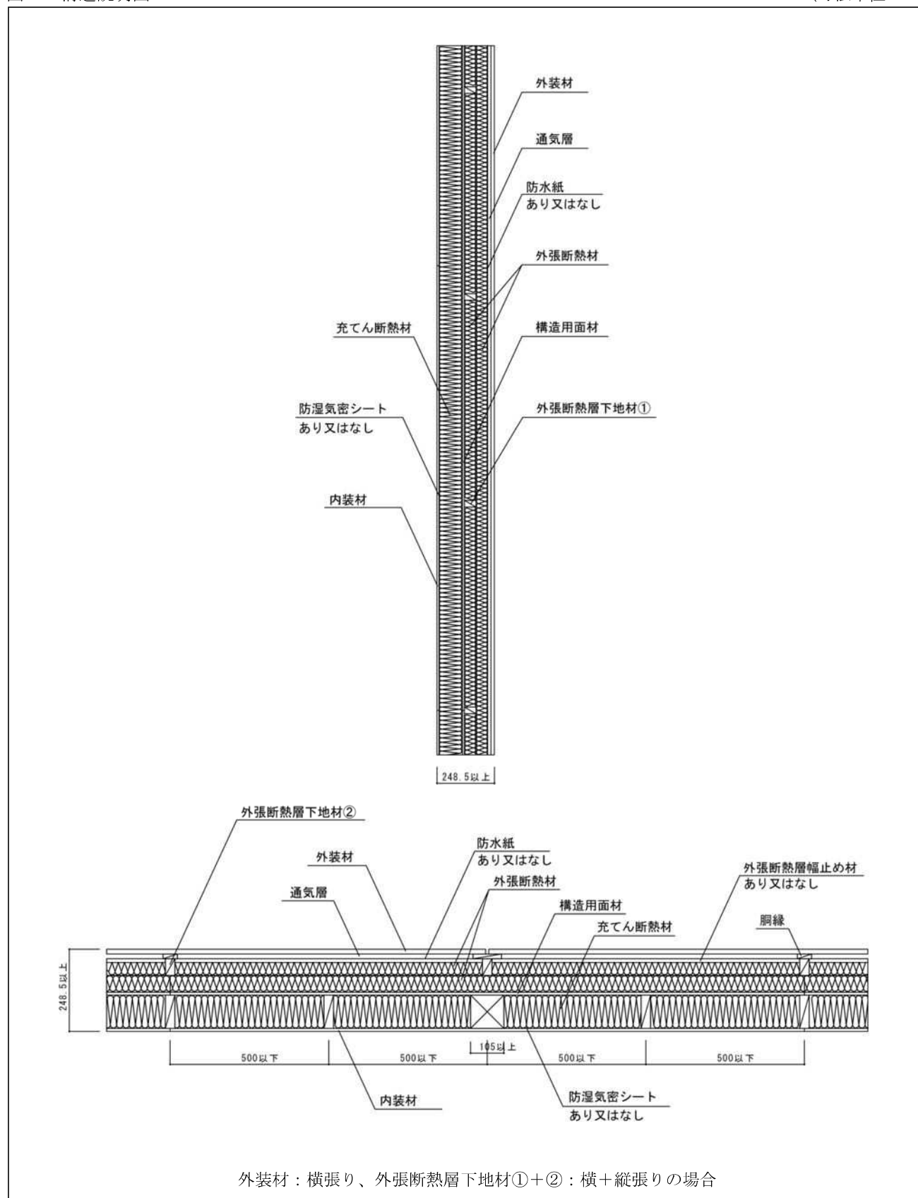
図4 構造説明図
