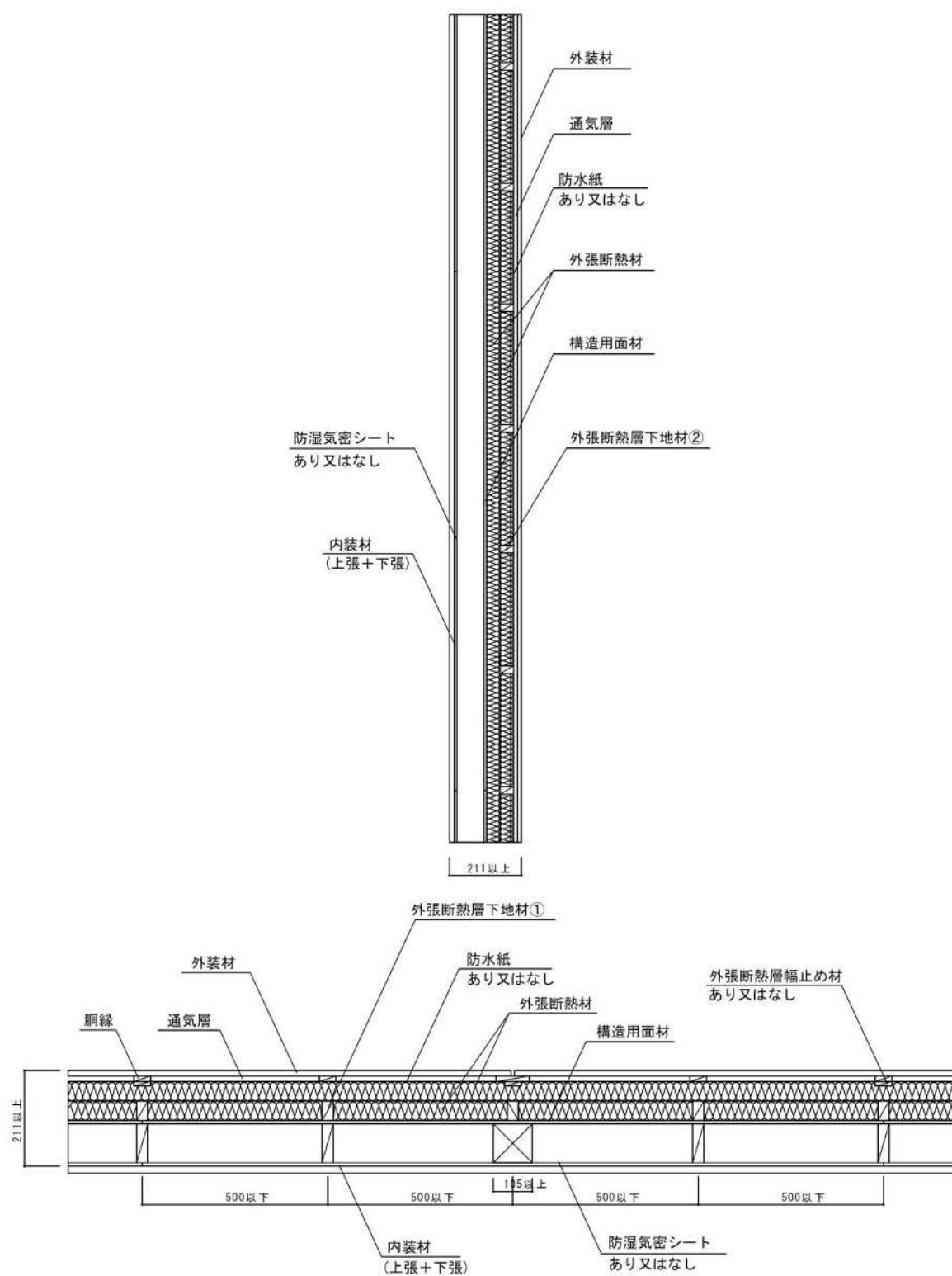
図5 構造説明図
