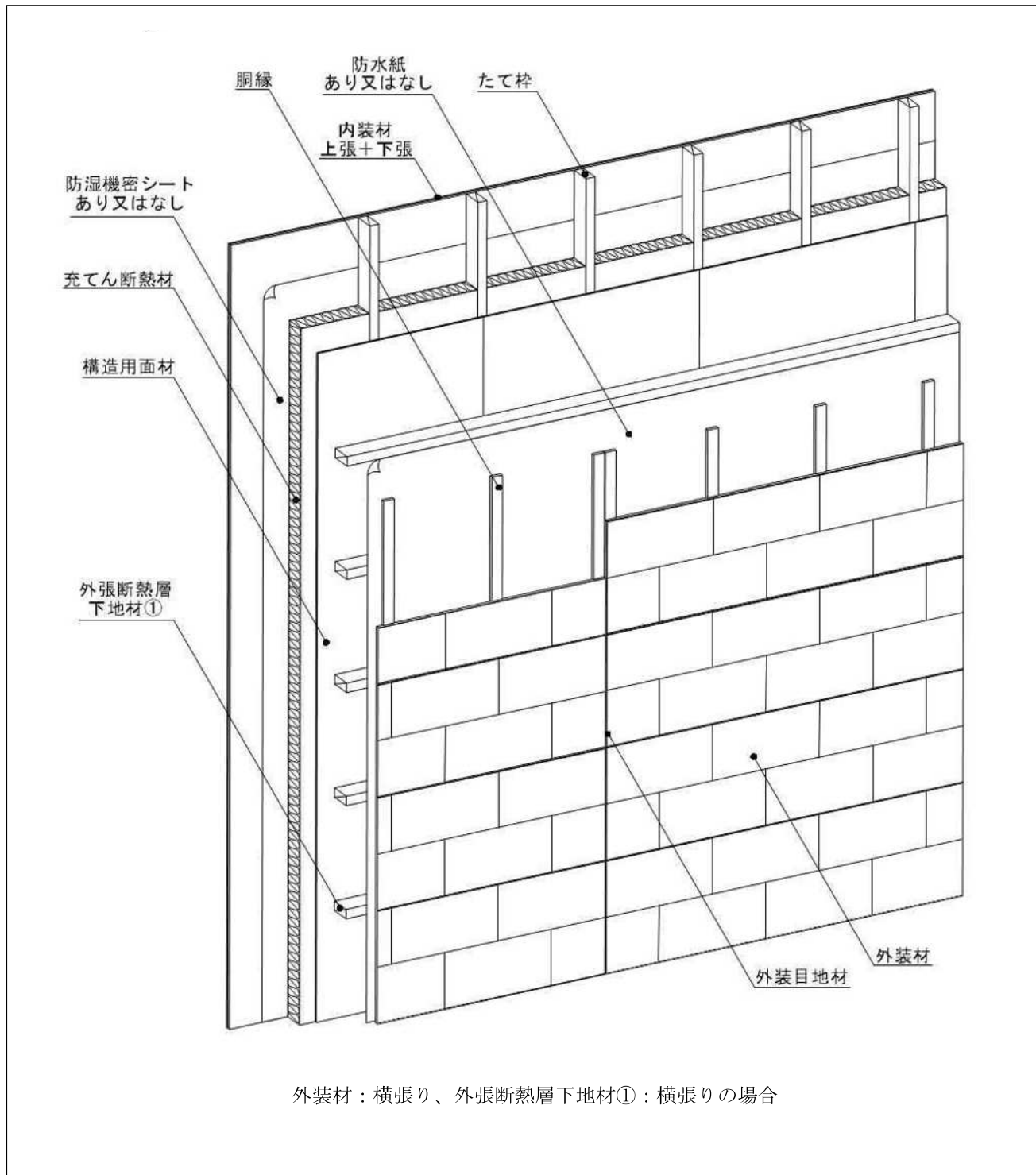
図1 構造説明図
