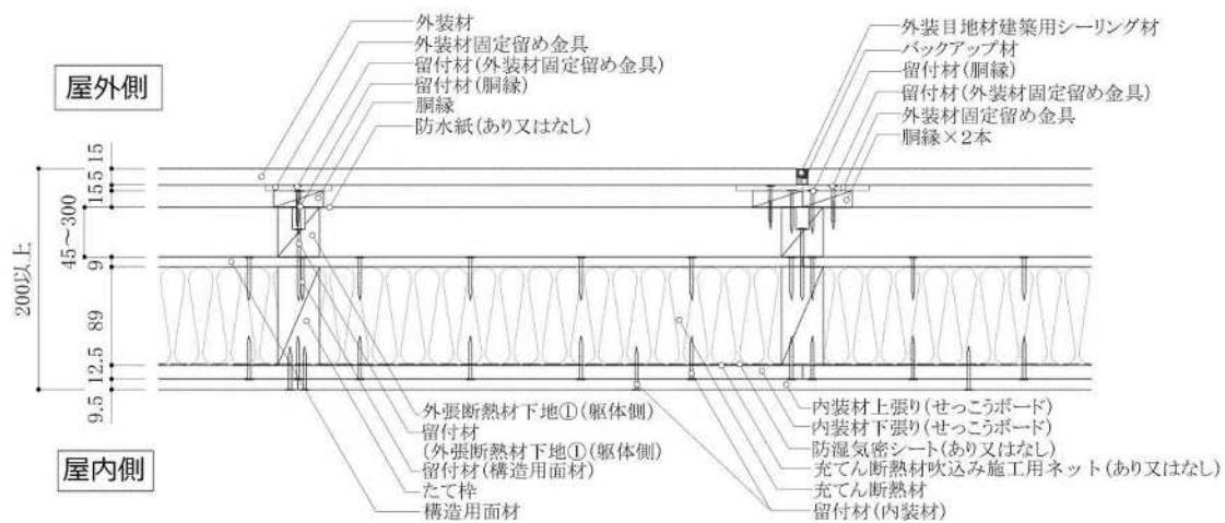
水平断面詳細図
