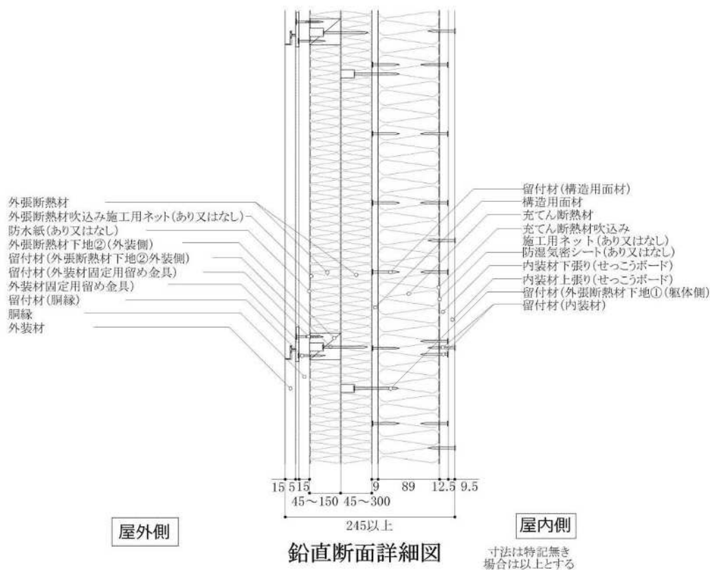
図 5 構造説明図
