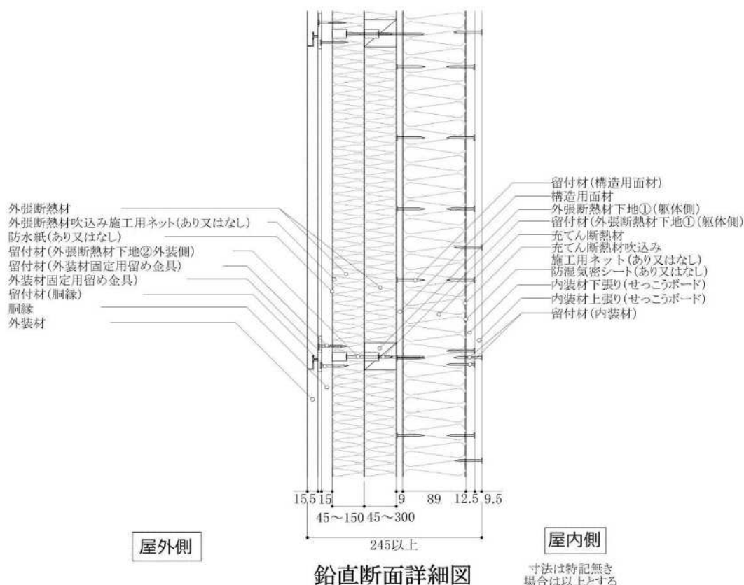
図4 構造説明図
