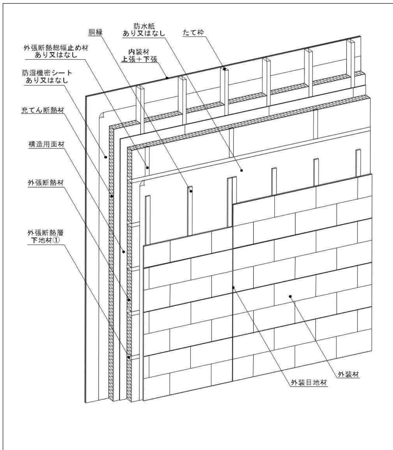
図1 構造説明図
