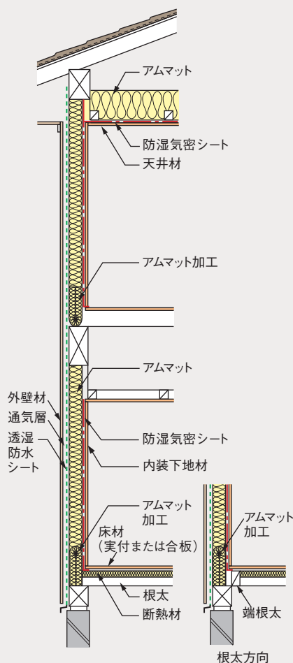
外壁(真壁)の場合
